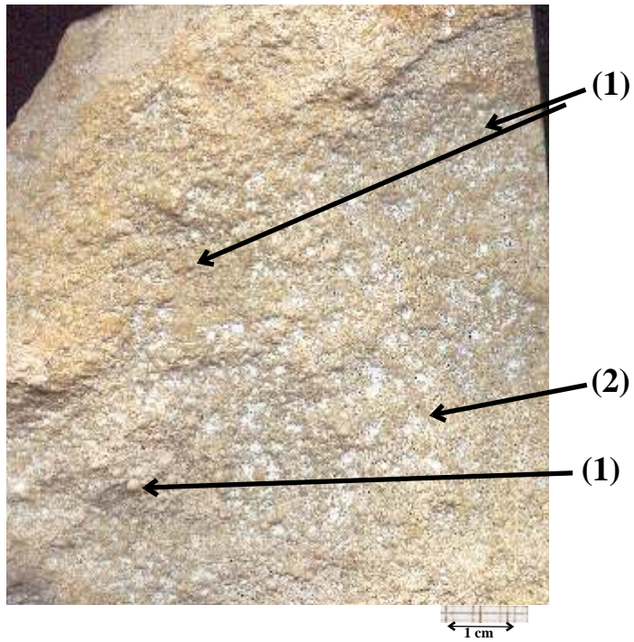
104_1 : Calcaire oolithique
